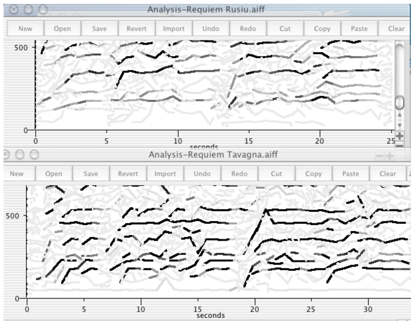
Figure 1 : Images obtenues avec le logiciel Spear ; extrait « Te decet hymnus », Rusiu, 0'54" à 1'19" — Tavagna extrait 1'17" à 1'51"
