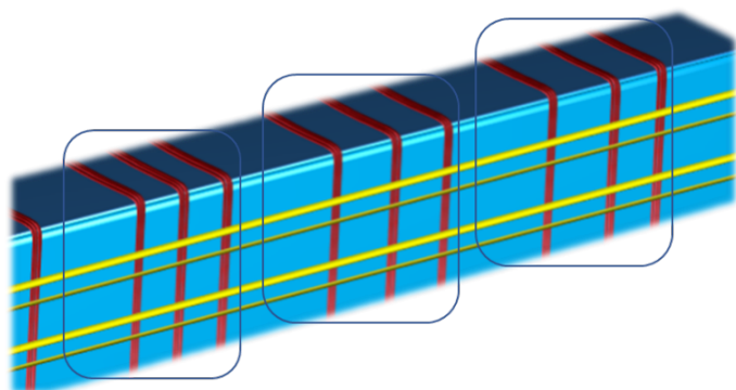
Schéma 2 : frettage du buzouq selon la pratique syrienne
